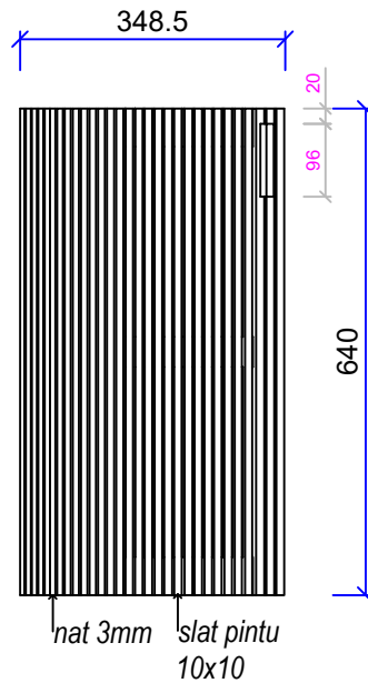
FRONT VIEW T. Depan pintu
