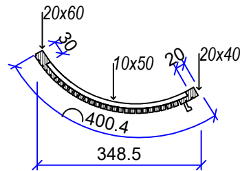
TOP VIEW T. Atas pintu
