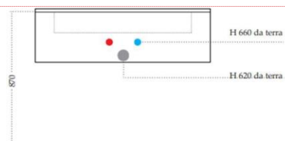
UNTERBAUTEN 90 mit integriertem Waschbecken
